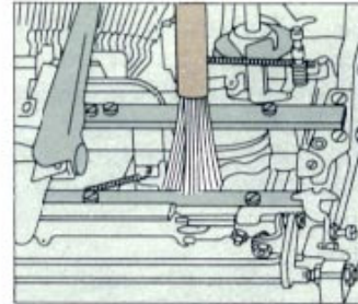
A kocsi szerkezet szeparátorát portalanítsuk ecsettel.
