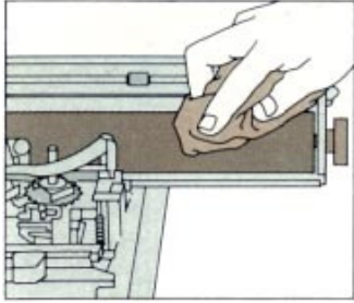
A gumihenger tisztítása puha alkoholos kendővel történik.
