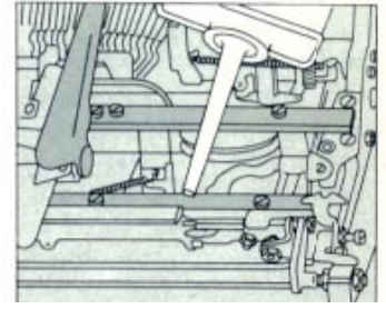
A szeparátort finom műszerolajjal olajozzuk meg.
