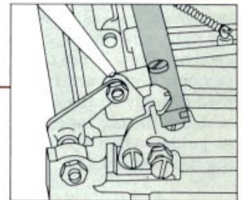
Olajozzuk meg a forgó alkatrészeket.
